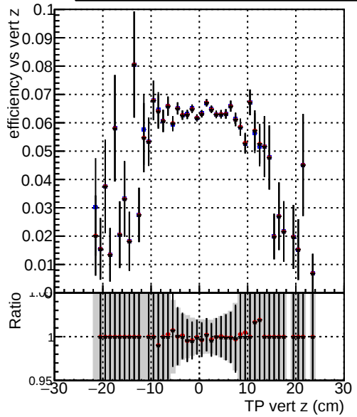
Efficiency vs. TP vert z (cm) —●— DQM_TT_CKF_ORIG —●— DQM_TT_CKFlowPIT_ORIG —●— DQM_TT_CKFlowPIT_MODIF
