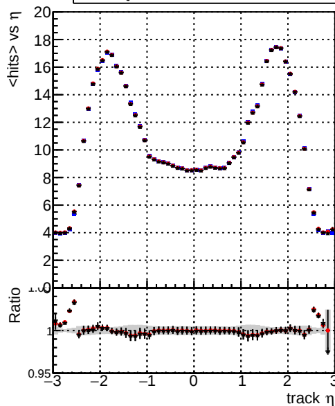
mean hits vs \eta — DQM_TT_CKF_ORIG — DQM_TT_CKFlowPIT_ORIG — DQM_TT_CKFlowPIT_MODIF
