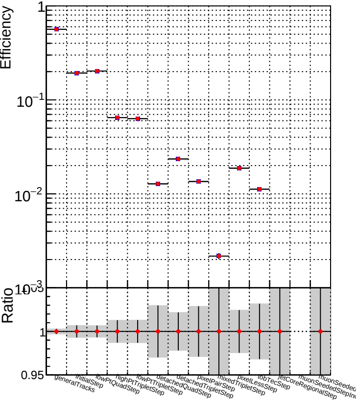
DQM_TT_CKF_ORIG DQM_TT_CKF_MODIF
