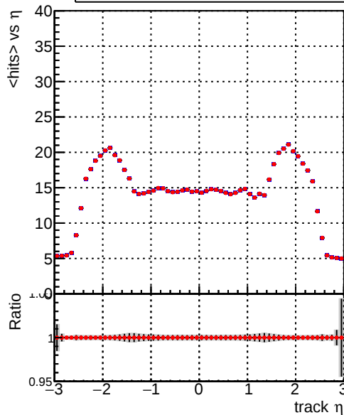
— DQM_TT_CKF_ORIG — DQM_TT_CKF_MODIF
