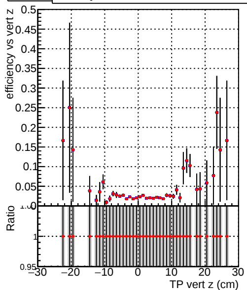
Efficiency vs. TP vert z (cm) — DQM_TT_CKF_ORIG — DQM_TT_CKF_MODIF
