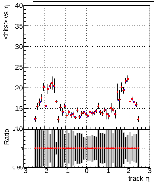
mean hits vs \eta — DQM_TT_CKF_ORIG — DQM_TT_CKF_MODIF
