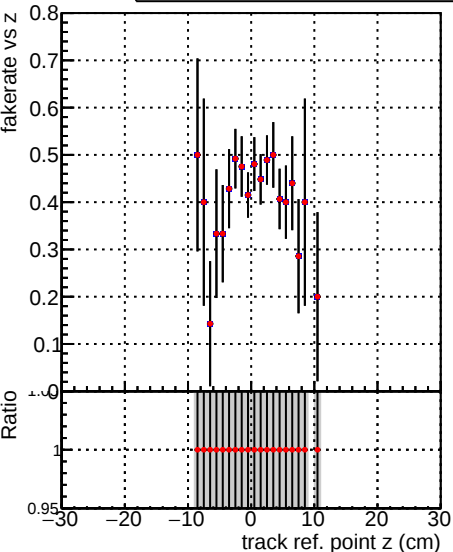
Fake rate vs v DQM_TT_CKF_ORIG DQM_TT_CKF_MODIF
