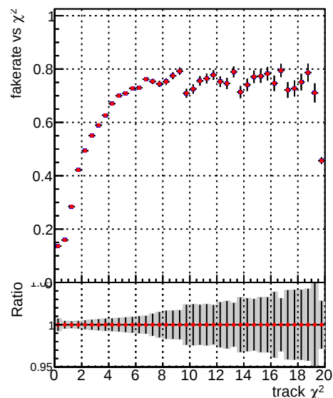
Fake rate vs. — DQM TT CKF ORIG — DQM TT CKF MODIF
