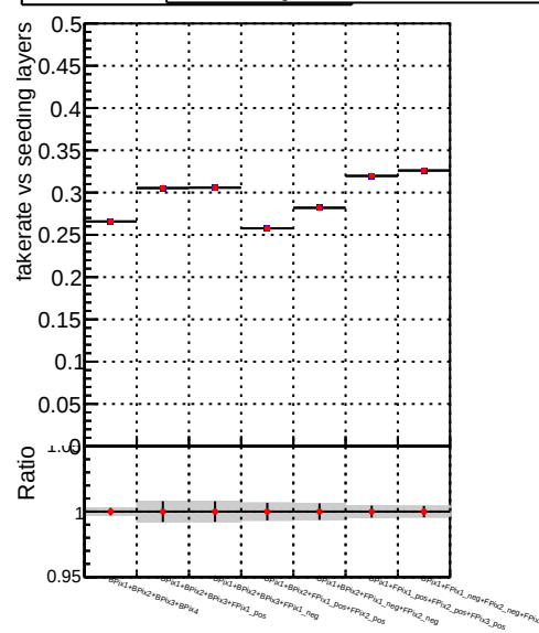
Fake rate vs. — DQM TT CKF ORIG — DQM TT CKF MODIF
