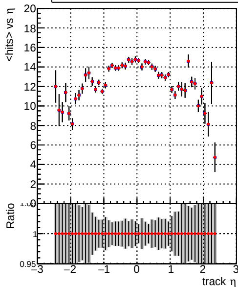
mean hits vs \eta — DQM_TT_CKF_ORIG — DQM_TT_CKF_MODIF
