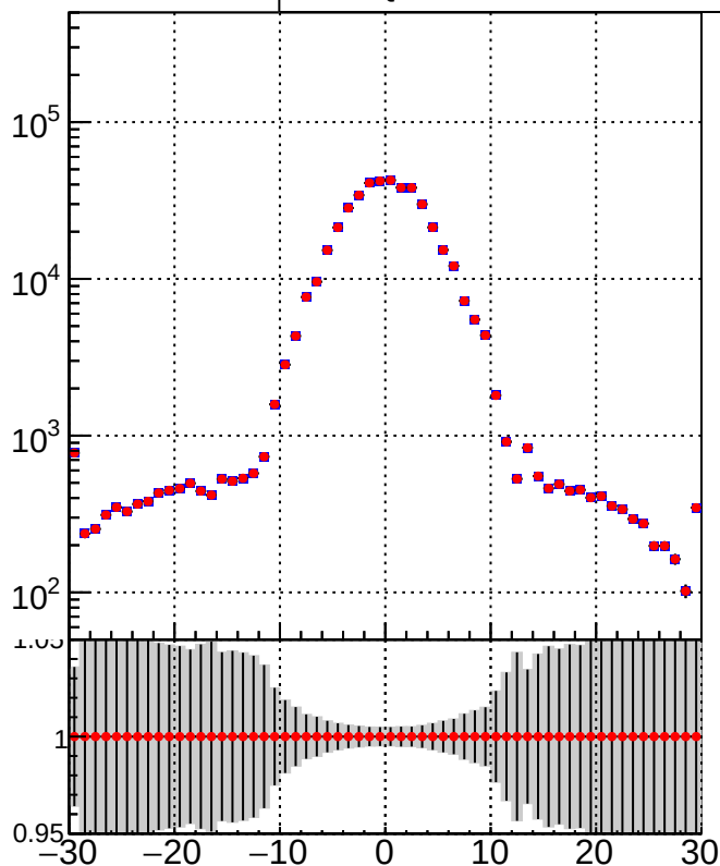
DQM_TT_mkFit_
