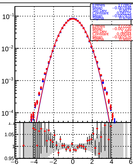
RecoAllAssoc2GenMatched_PulIZ
