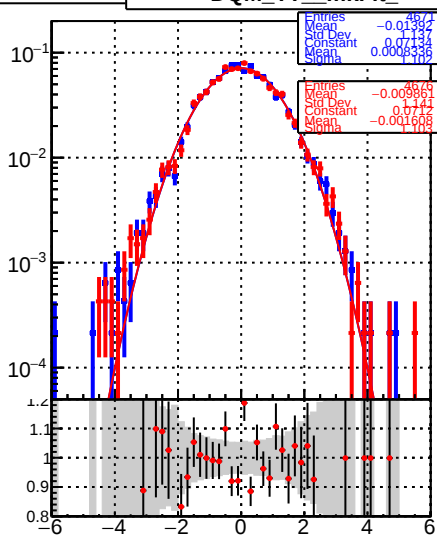
RecoPVAssoc
