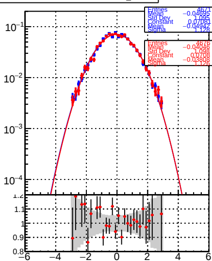
RecoPVAssoc2GenPVMatched_PulIZ
