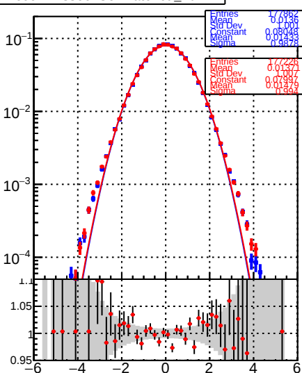
RecoAllAssoc2GenMatched_PulIX
