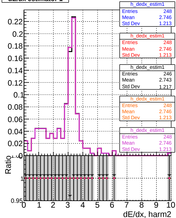
dE/dx estimator 1
