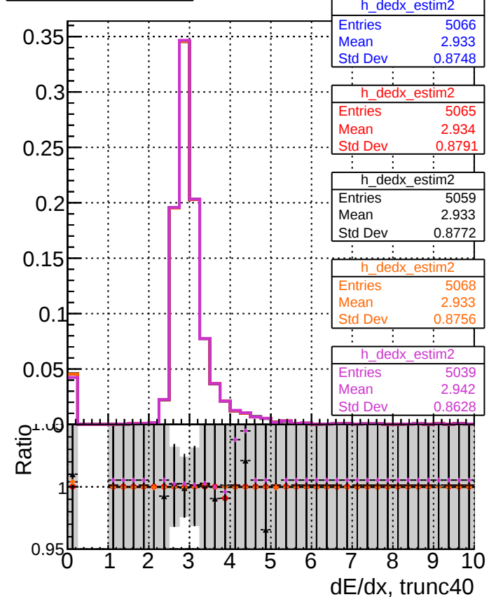
dE/dx estimator 2
