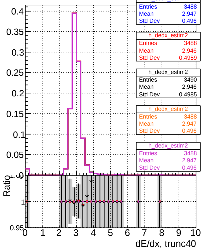
dE/dx estimator 2
