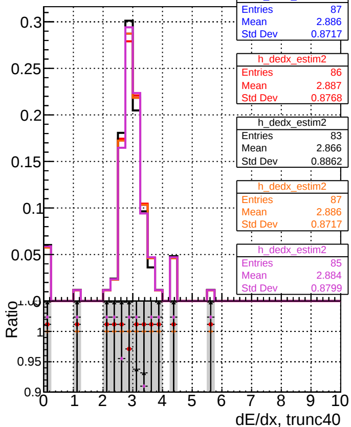
dE/dx estimator 2
