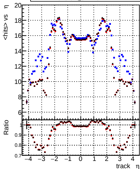
mean hits — CKFInit_CKFHPtT — mkFitInit_CKFHPtT — mkFitInitNoFit_CKFHPtT
