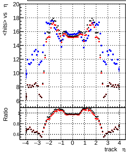
mean hits vs \eta — CKFInit_CKFHPtT — mkFitInit_CKFHPtT — mkFitInitNoFit_CKFHPtT
