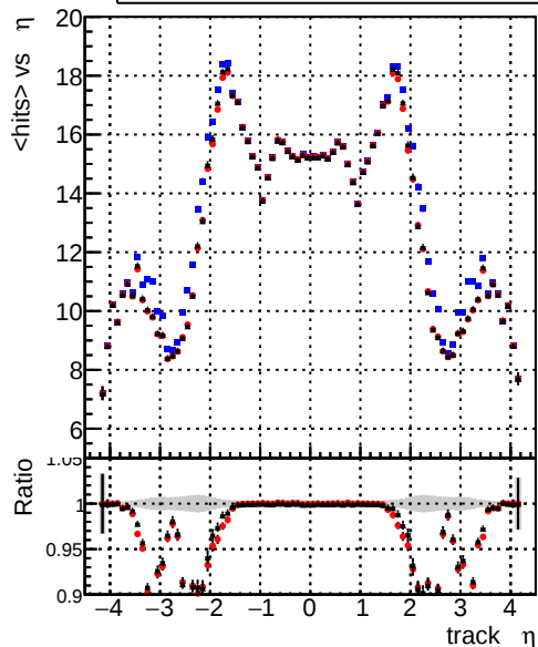
mean hits vs \eta CKFitInit_CKFHPtT mkFitInit_CKFHPtT mkFitInitNoFit_CKFHPtT
