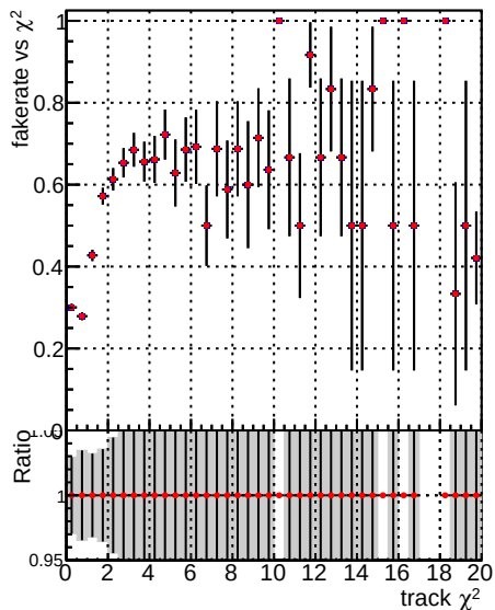
Fake rate vs. —•— DQM CKF TTbase —•— DQM CKF TTtest125xNEW
