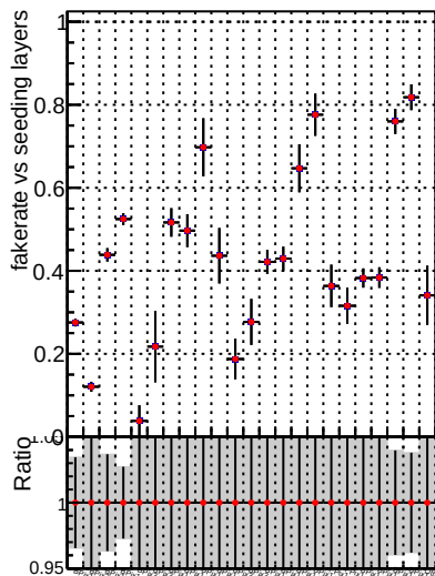
Fake rate vs. —•— DQM CKF TTbase —•— DQM CKF TTtest125xNEW
