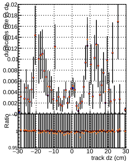
mal=mkFitNewDet33-RECO al=mkFitNewDetNoF-RECO
