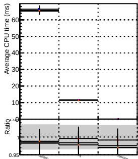
duplicateMerge
