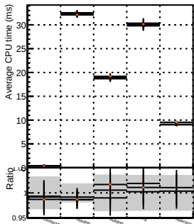
mixedTripletStep
