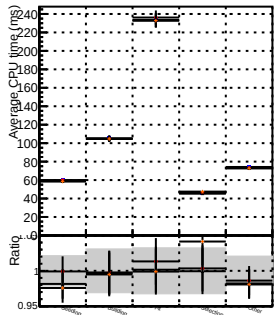
InitialStep
