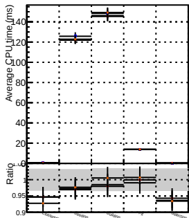
ConvStep
