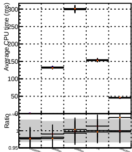
lowPTTripletStep
