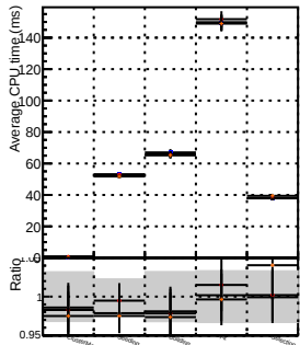
highPTTripletStep
