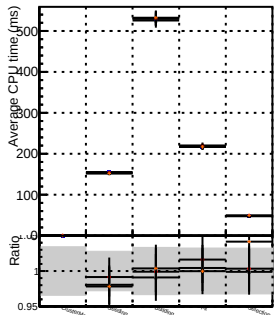
lowPTQuadStep
