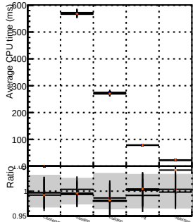
pixelLessStep
