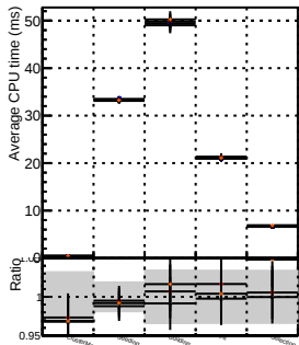
pixelPairStep
