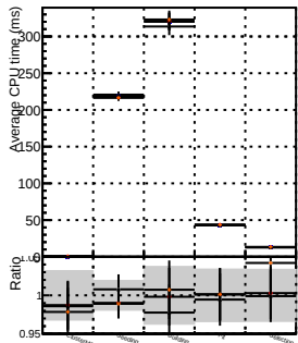
tobTecStep
