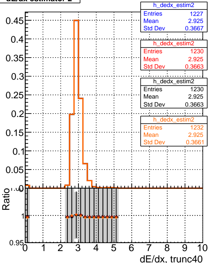
dE/dx estimator 2
