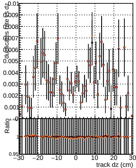
al=mkFitNewDet33-RECO al=mkFitNewDetNOF-RECO
