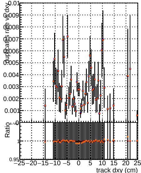
al=mkFitNewDet33-RECO al=mkFitNewDetNOF-RECO
