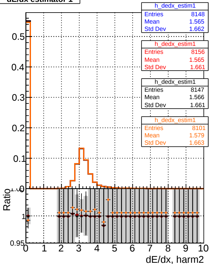
dE/dx estimator 1
