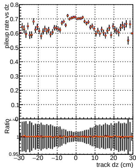
z = 0.8
