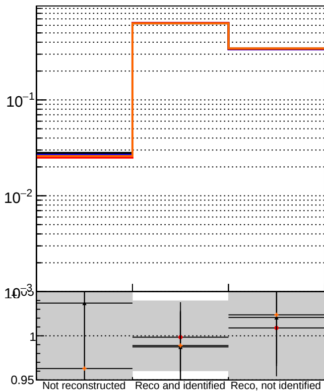
DQM_DisplacedSUSY_CKF_ DQM_DisplacedSUSY_mkFit_ DQM_DisplacedSUSY_CKF_BDT_ DQM_DisplacedSUSY_mkFit_BDT_
