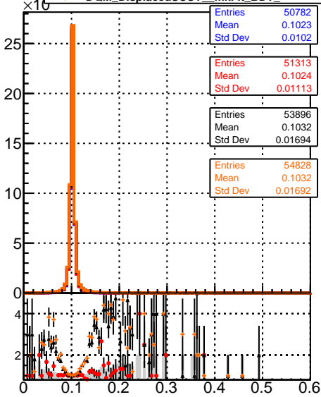
Recons DQM_DisplacedSUSY CKF DQM_DisplacedSUSY mkFit DQM_DisplacedSUSY CKF_BDT DQM_DisplacedSUSY mkFit_BDT
