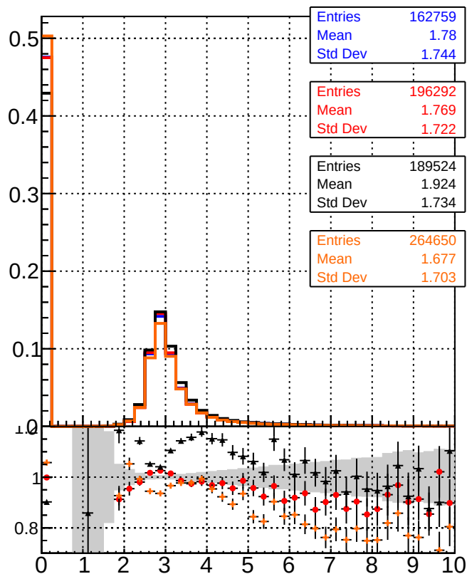
dE/dx estimator 2
