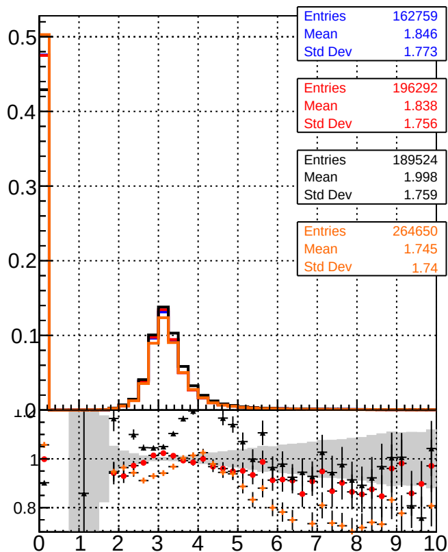
dE/dx estimator 1
