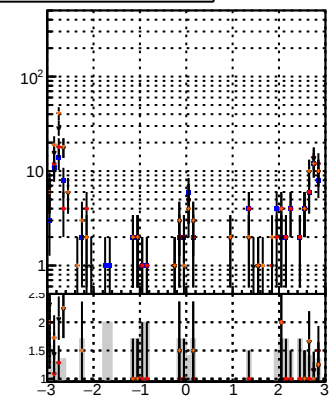
N of reco track vs \eta 95 eta
