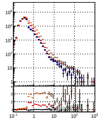
N of reco track vs \eta 95 eta
