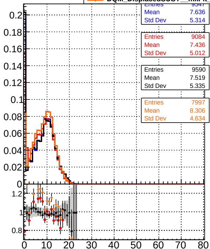
— DQM_DisplacedSUSY_CKF — DQM_DisplacedSUSY_mkFit — DQM_DisplacedSUSY_CKF_BDT — DQM_DisplacedSUSY_mkFit_BDT
