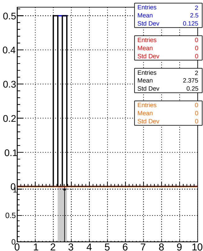
dE/dx estimator 2
