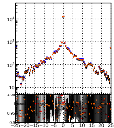
N of sim DQM_DisplacedSUSY_CKF_ DQM_DisplacedSUSY_mkFit_ DQM_DisplacedSUSY_CKF_BDT_ DQM_DisplacedSUSY_mkFit_BDT_
