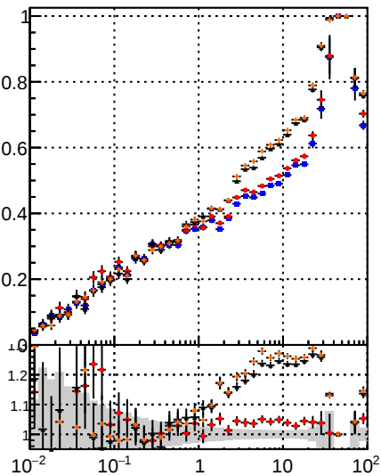
Fake rate vs v —■— DOM —■— CKE —★— DOM —★— CKE —×— DOM —×— BDT —★— DOM —★— mktFit
