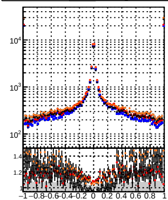
—●— DQM TT CKE fit —●— DQM TT CKE fit —●— DQM TT CKE fit —●— DQM TT CKE fit
