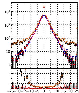
—●— DQM TT CKE fit —●— DQM TT CKE fit —●— DQM TT CKE fit —●— DQM TT CKE fit
