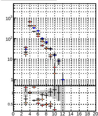
N of reco track vs 3D layer 0 0.00 1 0.00 2 0.00 3 0.00 4 0.00 5 0.00 6 0.00 7 0.00 8 0.00 9 0.00 10 0.00 11 0.00 12 0.00 13 0.00 14 0.00 15 0.00 16 0.00 17 0.00 18 0.00 19 0.00 20 0.00 21 0.00 22 0.00 23 0.00 24 0.00 25 0.00 26 0.00 27 0.00 28 0.00 29 0.00 30 0.00 31 0.00 32 0.00 33 0.00 34 0.00 35 0.00 36 0.00 37 0.00 38 0.00 39 0.00 40 0.00 41 0.00 42 0.00 43 0.00 44 0.00 45 0.00 46 0.00 47 0.00 48 0.00 49 0.00 50 0.00 51 0.00 52 0.00 53 0.00 54 0.00 55 0.00 56 0.00 57 0.00 58 0.00 59 0.00 60 0.00 61 0.00 62 0.00 63 0.00 64 0.00 65 0.00 66 0.00 67 0.00 68 0.00 69 0.00 70 0.00 71 0.00 72 0.00 73 0.00 74 0.00 75 0.00 76 0.00 77 0.00 78 0.00 79 0.00 80 0.00 81 0.00 82 0.00 83 0.00 84 0.00 85 0.00 86 0.00 87 0.00 88 0.00 89 0.00 90 0.00 91 0.00 92 0.00 93 0.00 94 0.00 95 0.00 96 0.00 97 0.00 98 0.00 99 0.00 100 0.00 101 0.00 102 0.00 103 0.00 104 0.00 105 0.00 106 0.00 107 0.00 108 0.00 109 0.00 110 0.00 111 0.00 112 0.00 113 0.00 114 0.00 115 0.00 116 0.00 117 0.00 118 0.00 119 0.00 120 0.00 121 0.00 122 0.00 123 0.00 124 0.00 125 0.00 126 0.00 127 0.00 128 0.00 129 0.00 130 0.00 131 0.00 132 0.00 133 0.00 134 0.00 135 0.00 136 0.00 137 0.00 138 0.00 139 0.00 140 0.00 141 0.00 142 0.00 143 0.00 144 0.00 145 0.00 146 0.00 147 0.00 148 0.00 149 0.00 150 0.00 151 0.00 152 0.00 153 0.00 154 0.00 155 0.00 156 0.00 157 0.00 158 0.00 159 0.00
