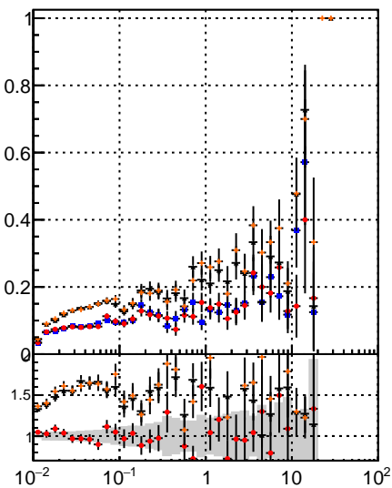
Fake rate vs \sqrt{z} —●— DQM IT CKE Fit —○— DQM IT CKE Fit —△— DQM IT BDT —□— DQM IT mkFit BDT
