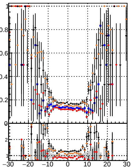
Fake rate vs d DQM IT GKE CKE DQM IT GKE BDT DQM IT GKE BDT
