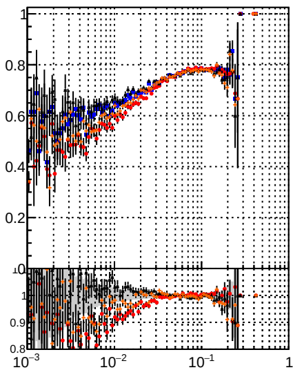
Fake rate vs \sqrt{s} Legend: DOM TT CKE BDT DOM TT CKE BDT DOM TT CKE BDT
