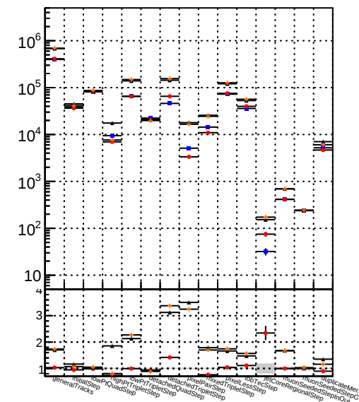
Number → DQM TT CKF BDT DQM TT mkFit BDT
