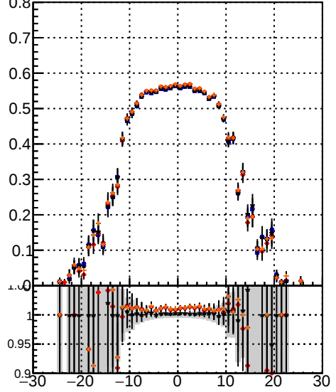
Efficiency vs. sim PV z —●— DQM TT CKF —◆— DQM TT mkFit —×— DQM TT CKF BDT —★— DQM TT mkFit BDT
