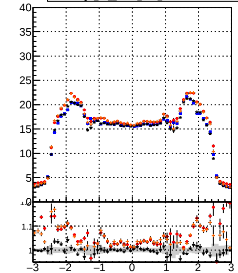
mean hit DQM TT CKF DQM TT mkFit DQM TT CKF BDT DQM TT mkFit BDT
