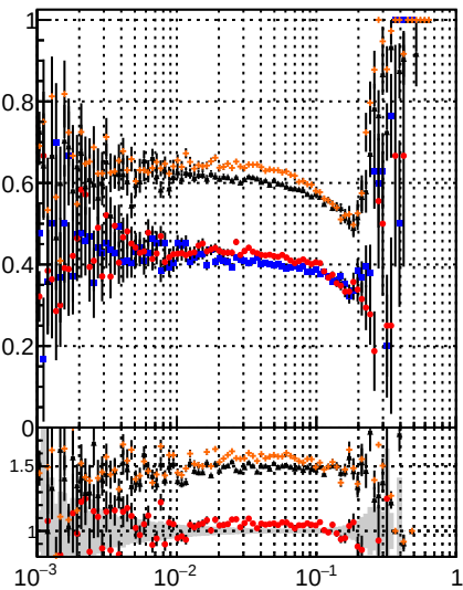
Fake rate vs \sqrt{s} DOM TT CKE CKE fit BDT DOM TT CKE CKE fit BDT DOM TT CKE CKE fit BDT
