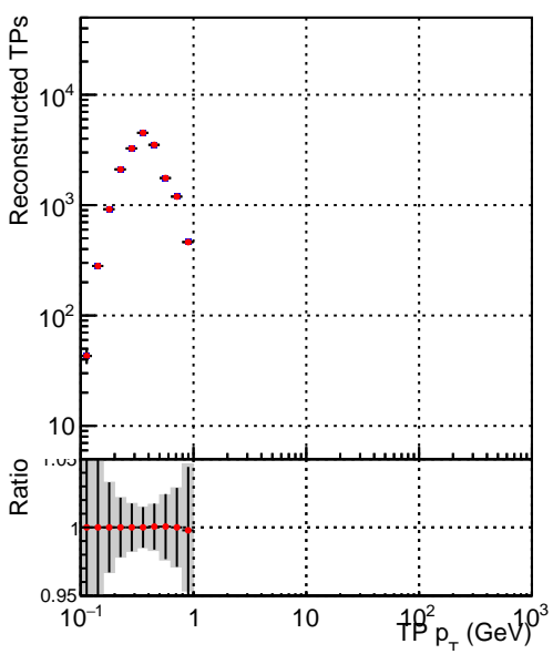
■ DQM_TT_ORIGINAL ● DQM_TT_MODIFIED_propToPlane_PRVersionFINAL6
