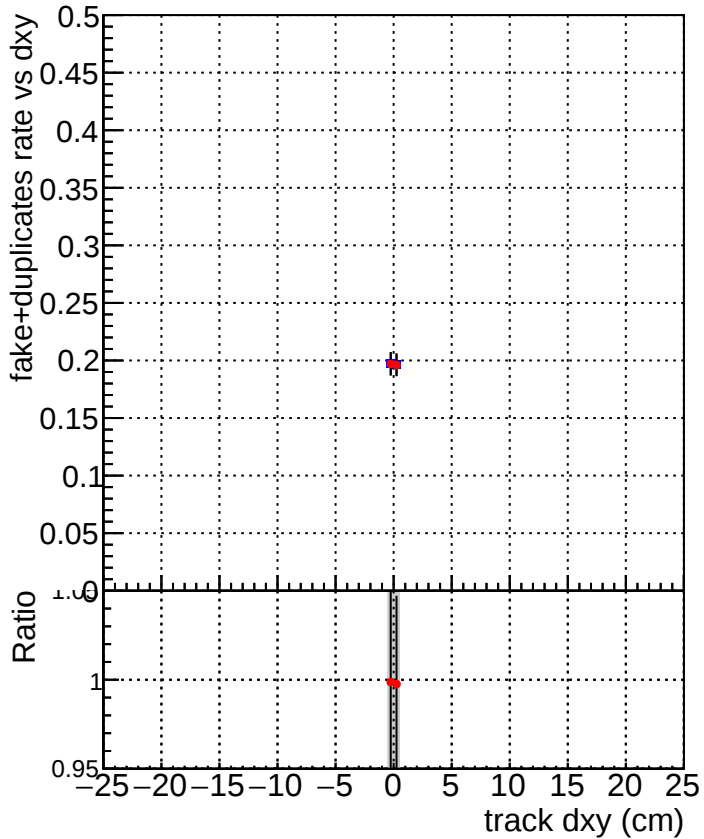
DQM_TT__ORIGINAL DQM_TT__MODIFIED_propToPlane_PRVersionFINAL6
