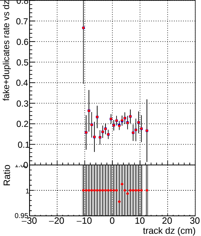
DQM_TT__ORIGINAL DQM_TT__MODIFIED_propToPlane_PRVersionFINAL6
