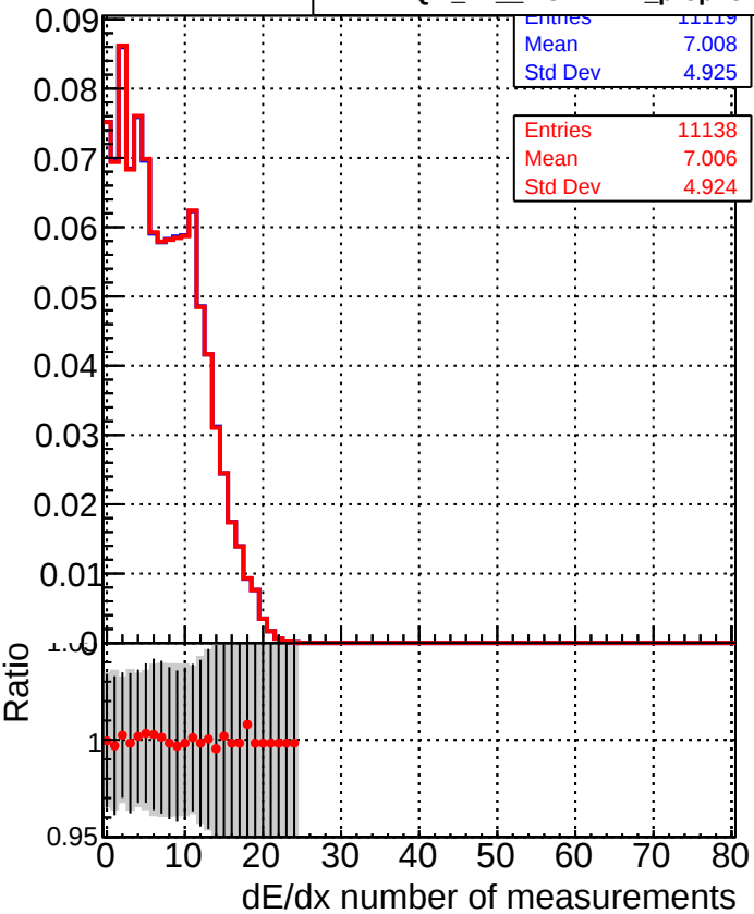
■ DQM_TT_ORIGINAL —●— DQM_TT_MODIFIED_propToPlane_PRVersionFINAL6
