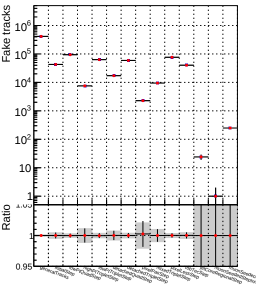
Number — DQM_TT_MODIFIED_propToPlane_PRVersionFINAL5
