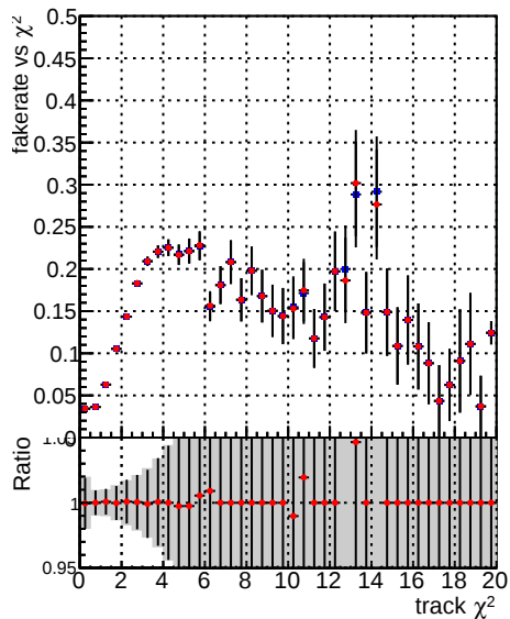
Fake rate vs. —●— DQM TT ORIGINAL —●— DQM TT MODIFIED_propToPlane_PRVersionFINAL5
