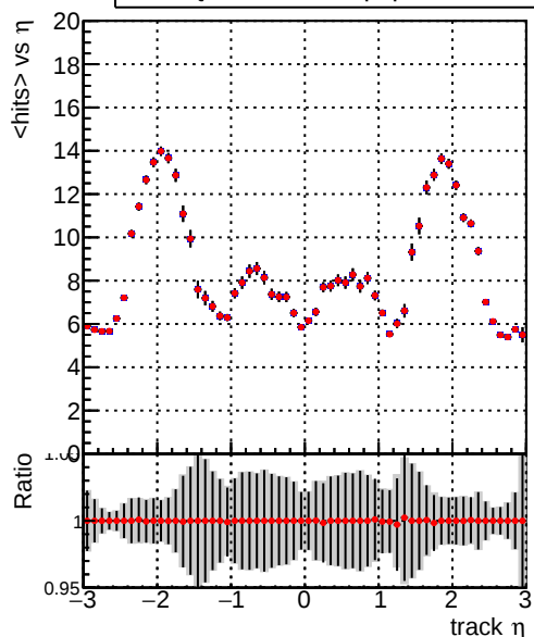
— DQM_TT_ORIGINAL — DQM_TT_MODIFIED_propToPlane_PRVersionFINAL5
