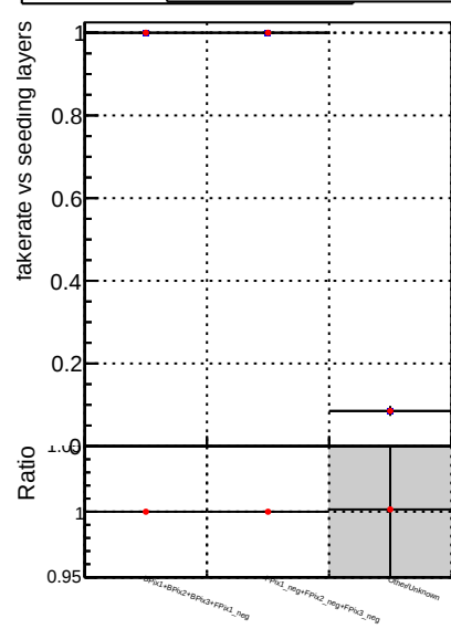
Fake rate vs. DQM TT ORIGINAL DQM TT MODIFIED propToPlane_PRVersionFINAL5
