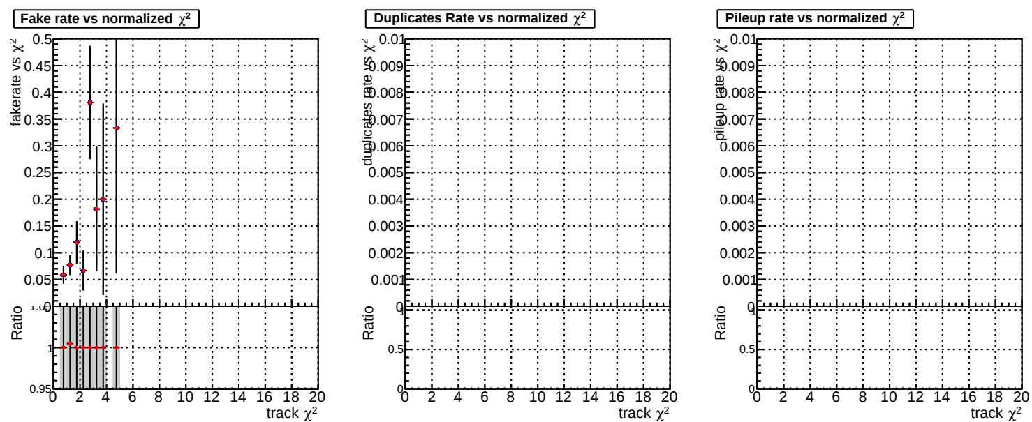
Fake rate vs. DQM TT ORIGINAL DQM TT MODIFIED propToPlane_PRVersionFINAL5
