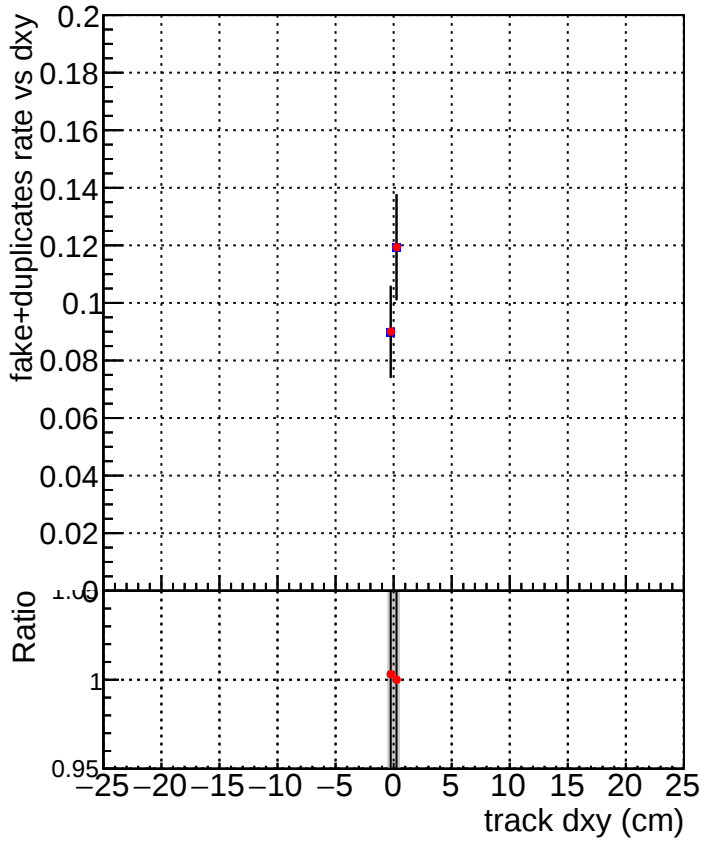
DQM_TT__ORIGINAL DQM_TT__MODIFIED_propToPlane_PRVersionFINAL5
