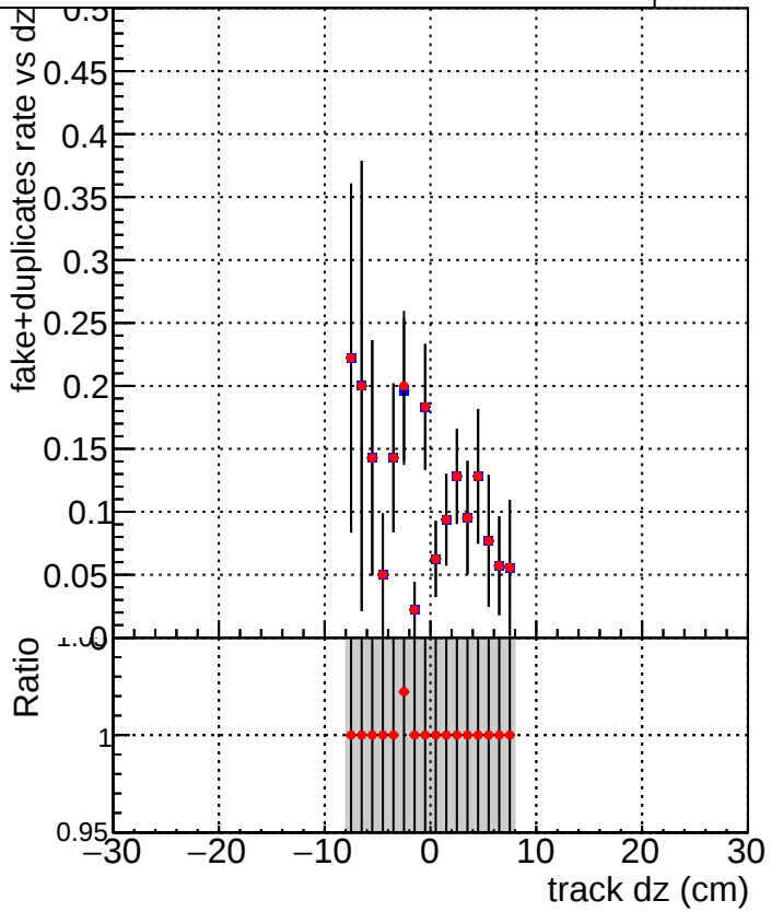
DQM_TT__ORIGINAL DQM_TT__MODIFIED_propToPlane_PRVersionFINAL5
